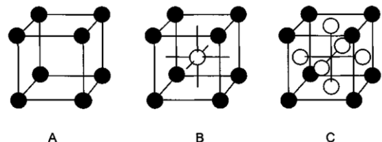
Fig. 14. Kubiske krystalsystemer. A: Det kubisk simple system. B: Det kubisk rumcentrerede system. C: Det kubisk fladecentrerede system.
